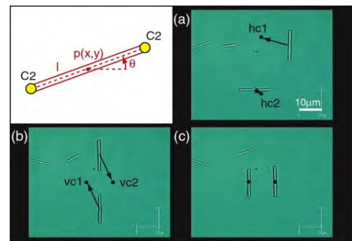
非球状な微小物 (四国センターで開発されたウイスカ) の自動操作の様子
